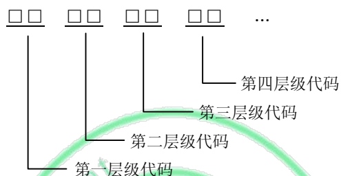
图1 代码结构图
